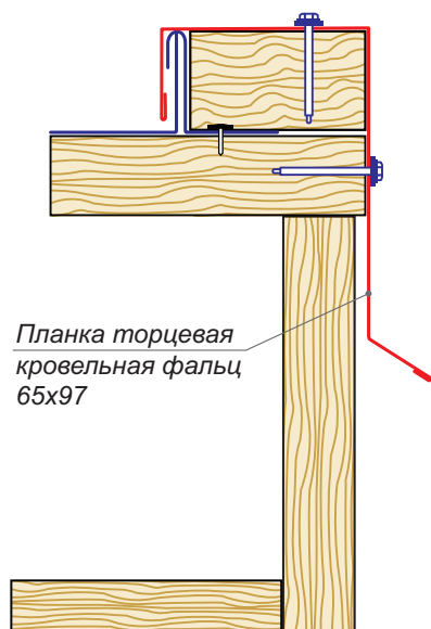
Кровля
