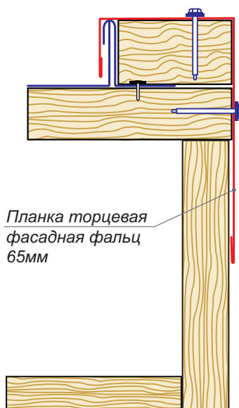
Фасад
